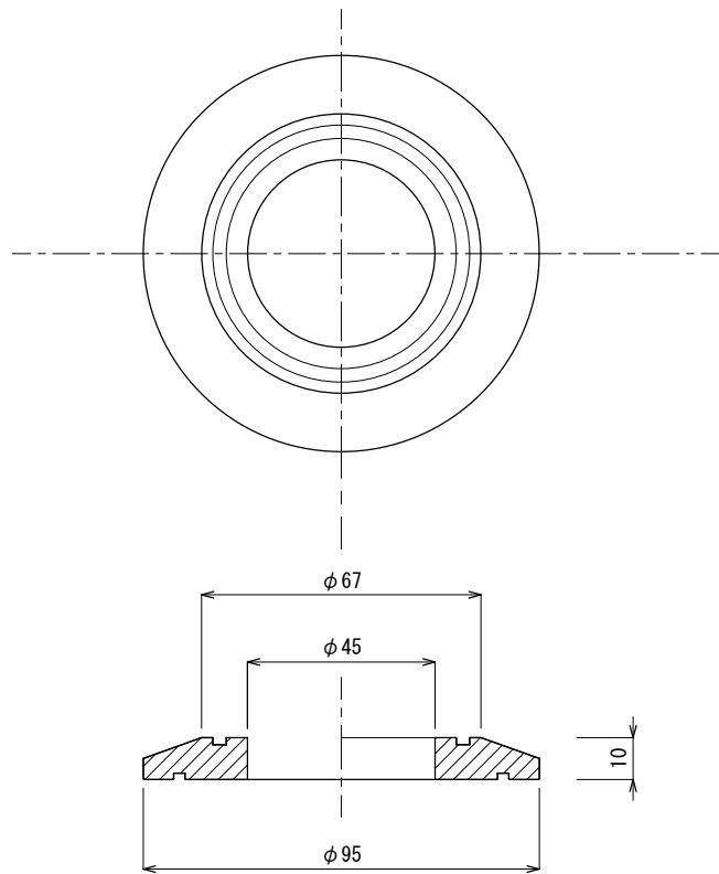
マウンティングディスク (スペーサー) L10.0 S=1/2
