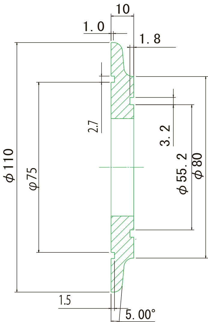
AA断面
