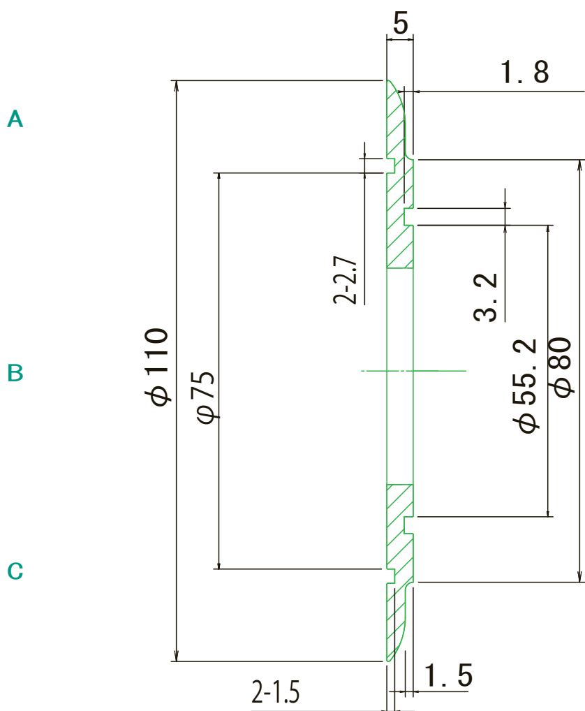
AA断面
